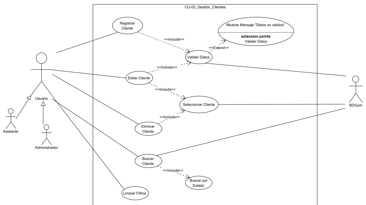
Figura 3: Diagrama detallado del caso de uso CU-03: Gestión de clientes
