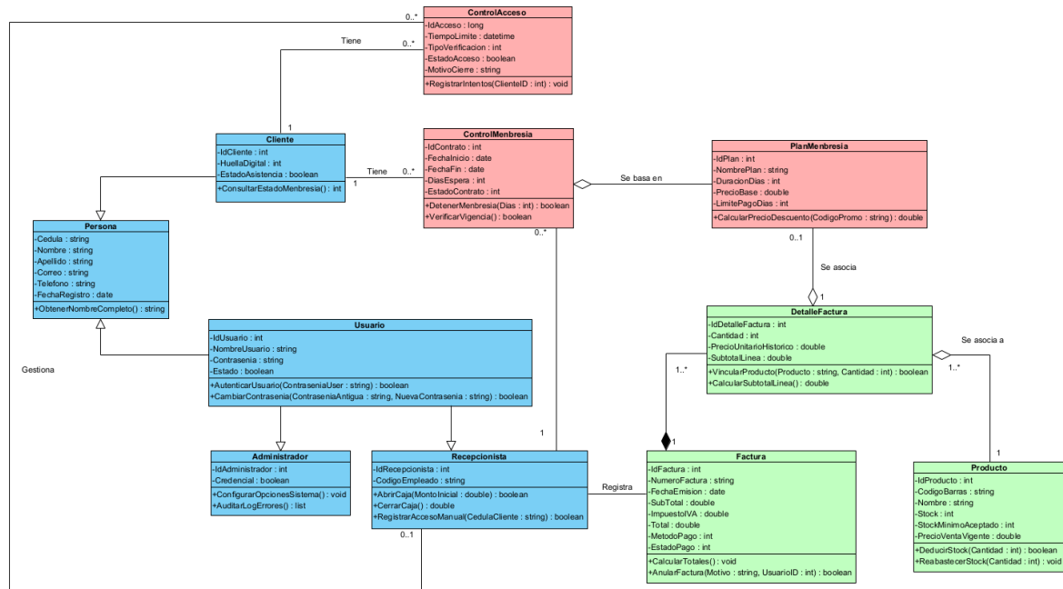
Figura 4: Diagrama de clases conceptual del dominio
