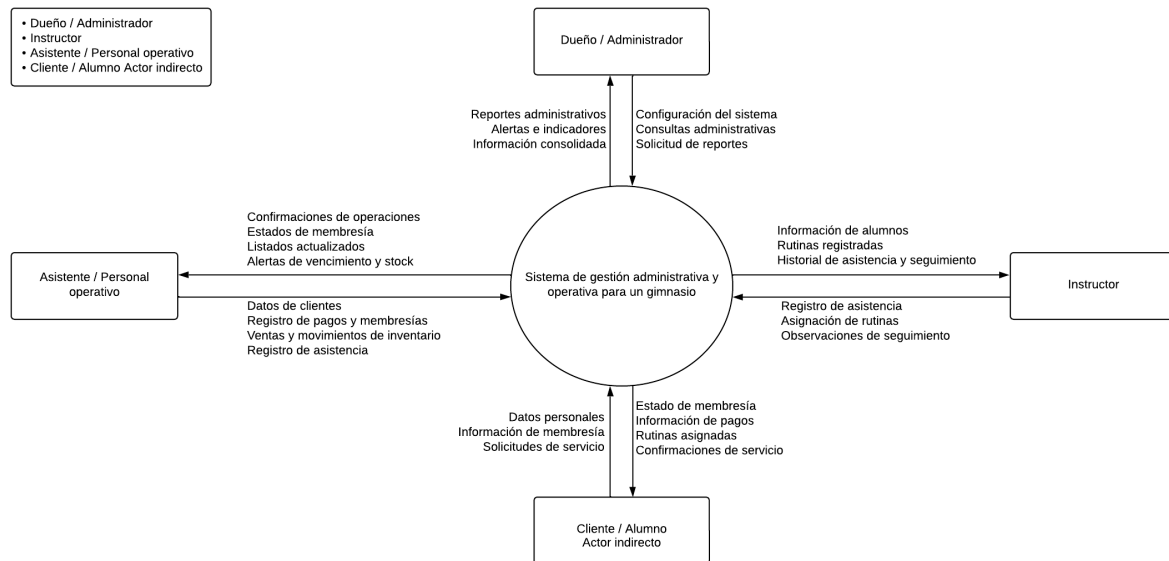
Figura 1: Diagrama de contexto del sistema objetivo
