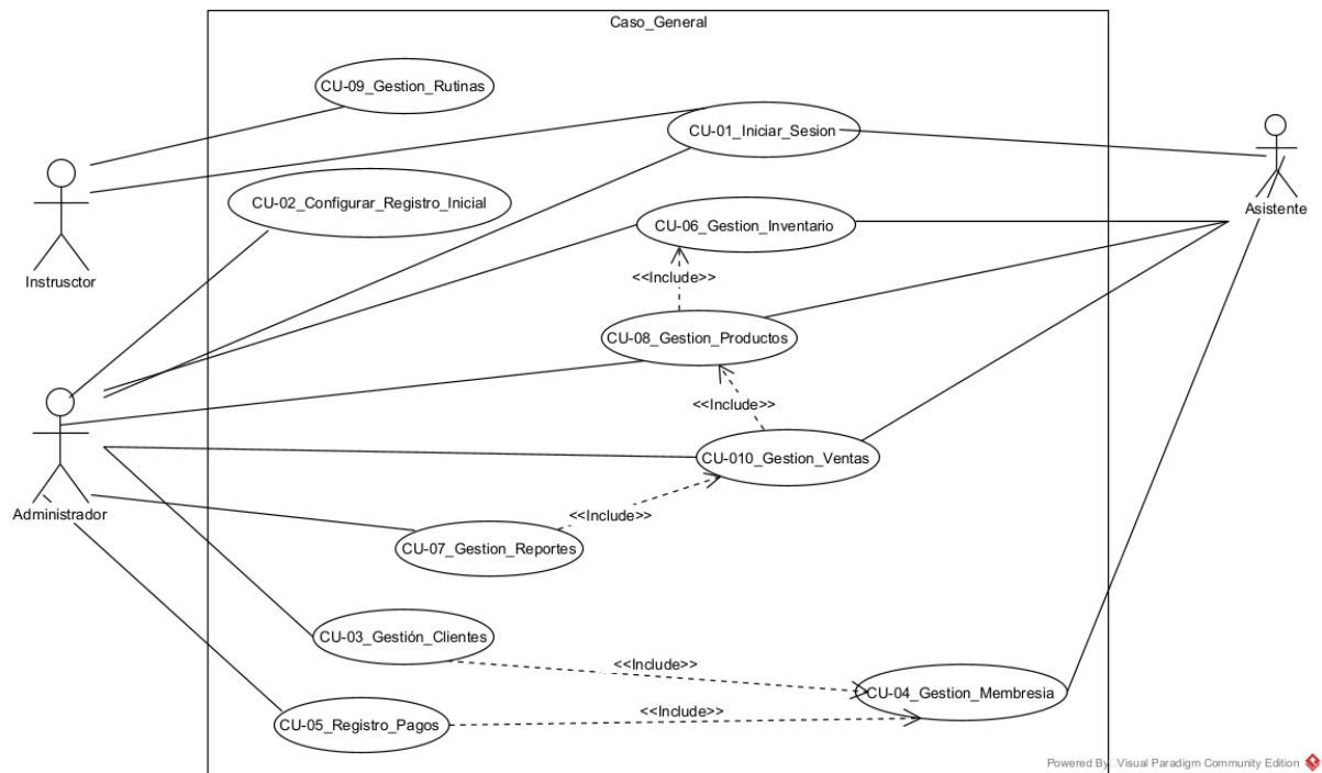
Figura 2: Diagrama general de casos de uso
